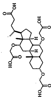
2a (CD 3 OOD/CDCl 3 , 500 MHz)
